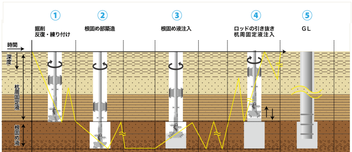
【杭工事の流れ】ハイブリッドニーディング工法（ドリルで掘削した穴に杭を建て込みます）
