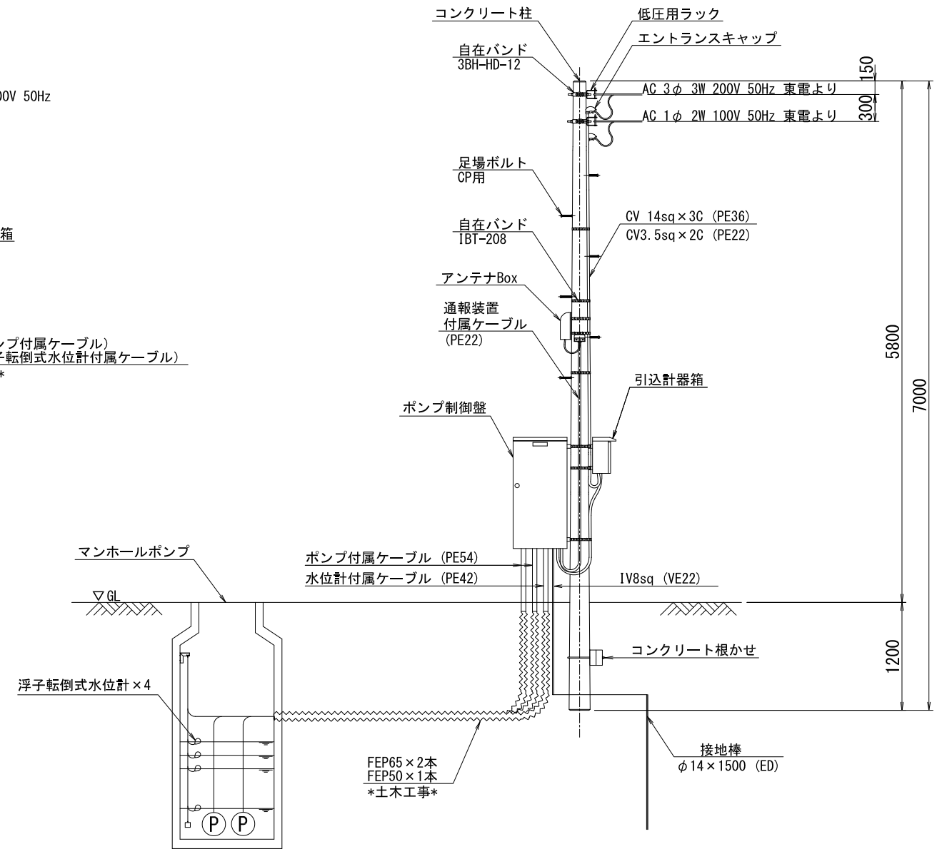
電力引込図 S=1/30
