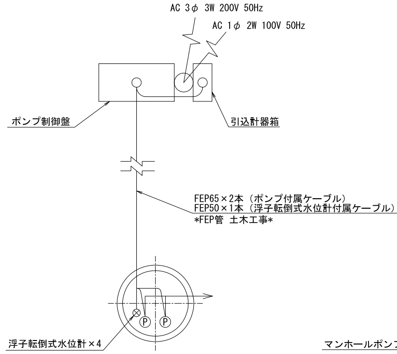
電力引込平面図
