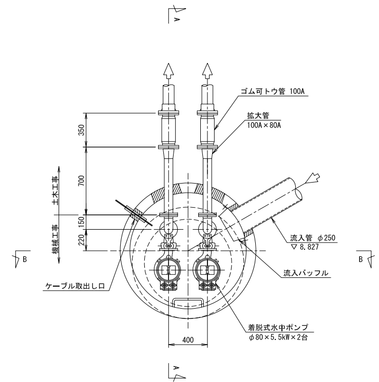
平面図 S=1/40
