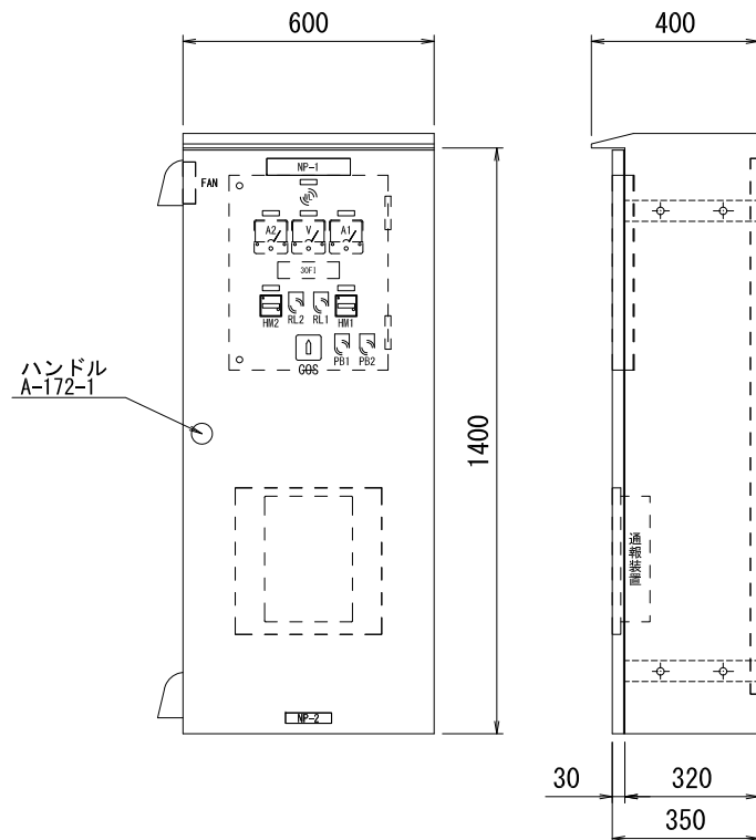
制御盤外形図 S=1/20
