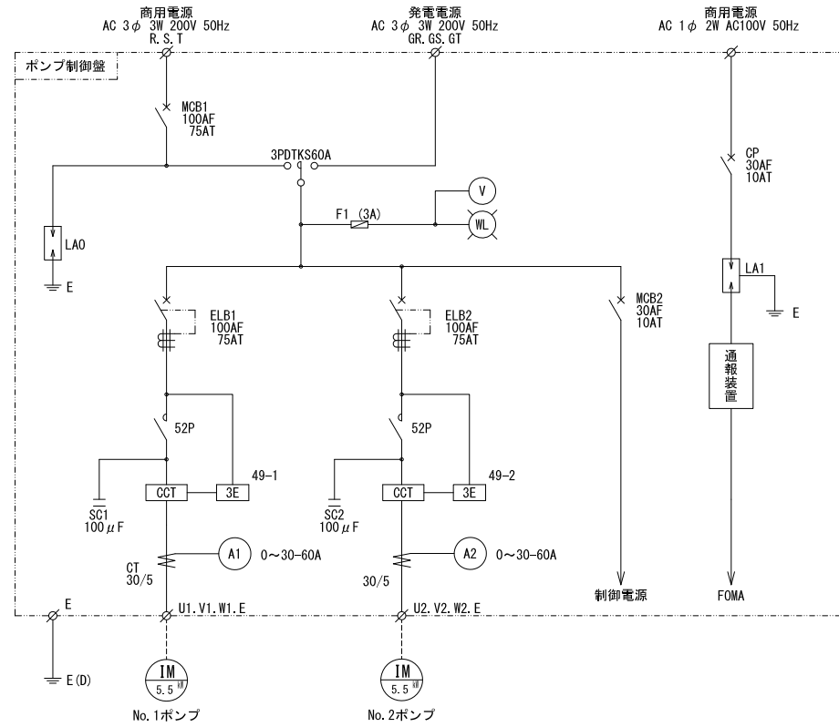
単線結線図
