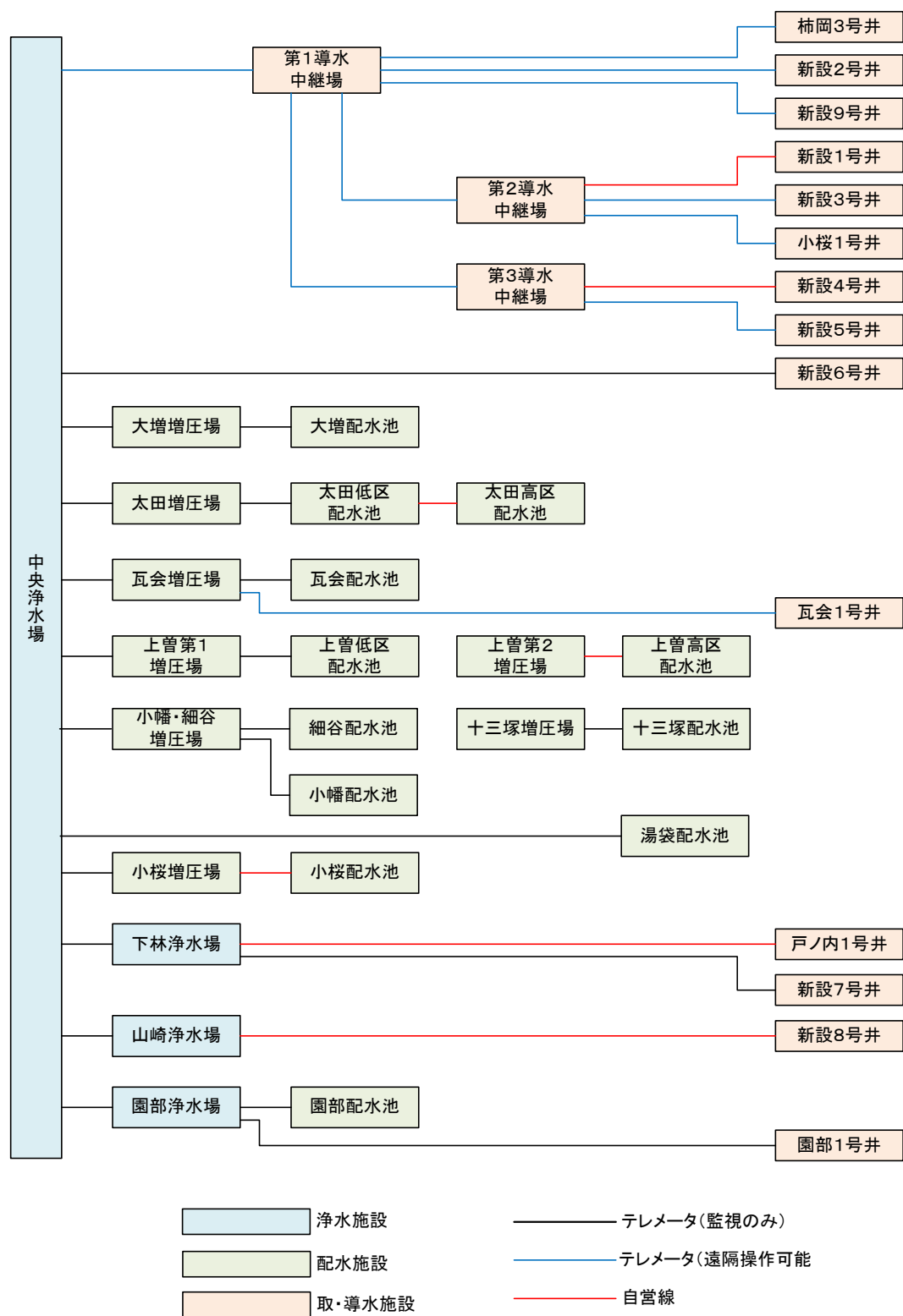
図 2-10 遠方監視系統図
