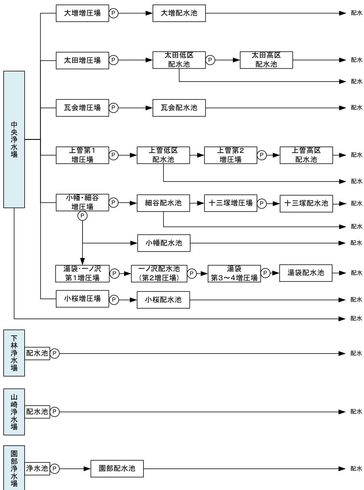
図 2-9 送水・配水施設フロー
