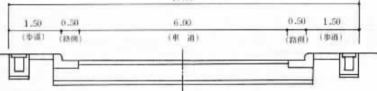
標準横断面図 S=1/100
