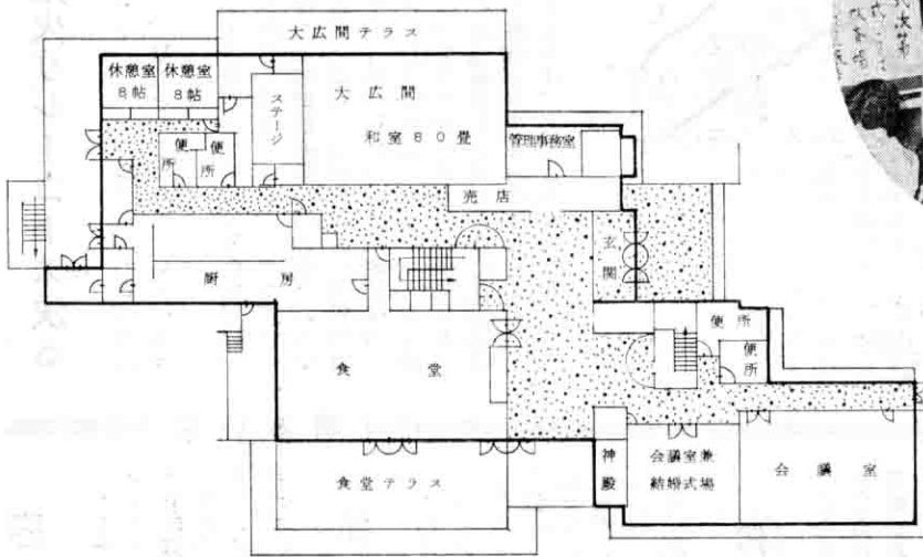
1階平面図
