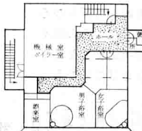
地下1階平面図
