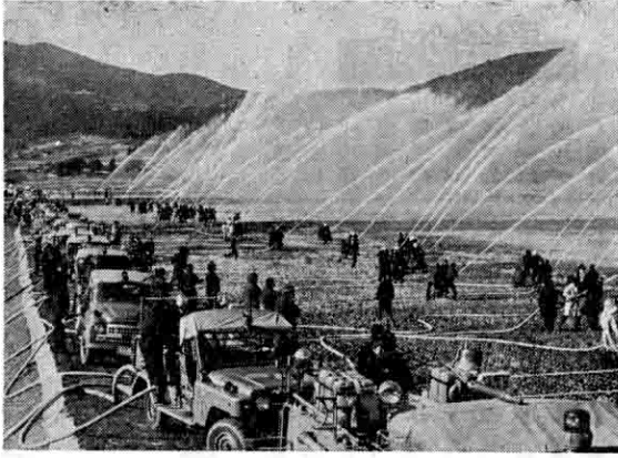
みごとな吉生小久保前でのいっせい放水試験
