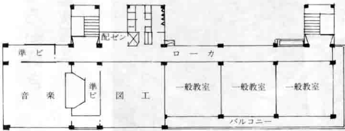
3階平面図
