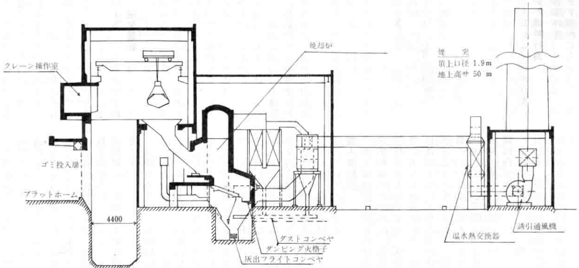
ゴミ処理場断面図
