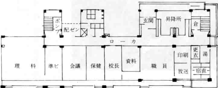
1階平面図
