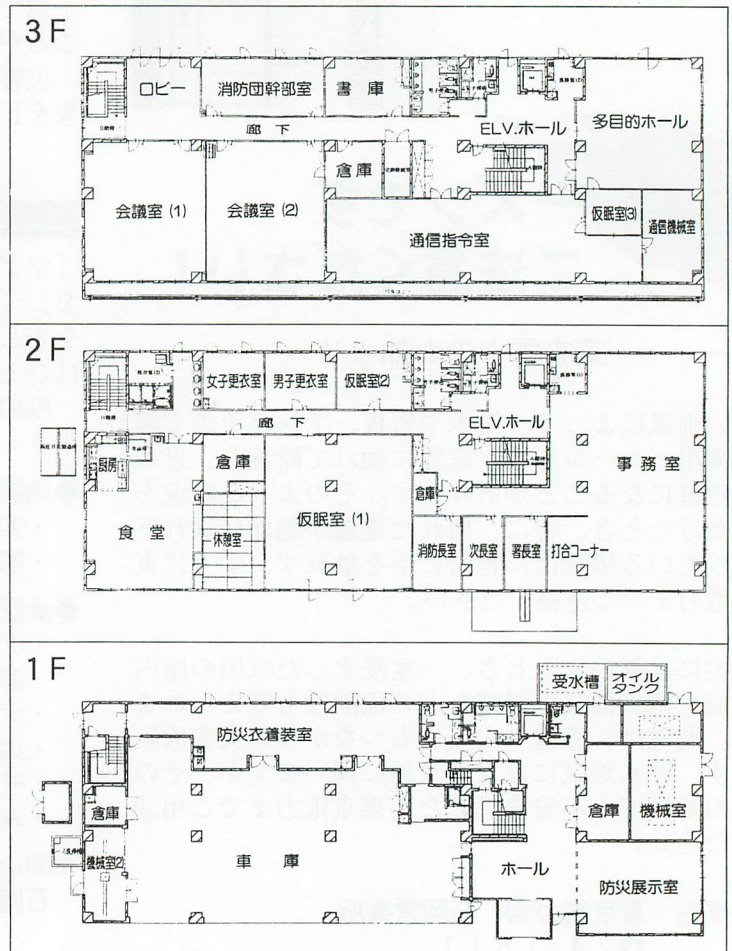
石岡市消防本部完成予想平面図
