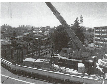
◆橋台部分の基礎工事
