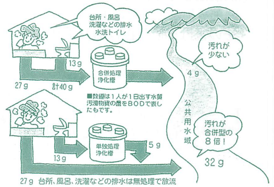
▲し尿と生活雑排水を処理できる合併処理浄化槽
