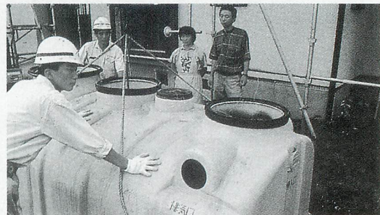
▲し尿と生活雑排水を処理できる合併処理浄化槽
