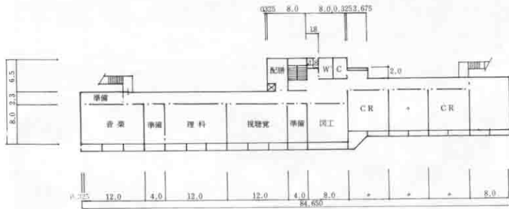
2階平面図
