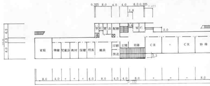
1階平面図
