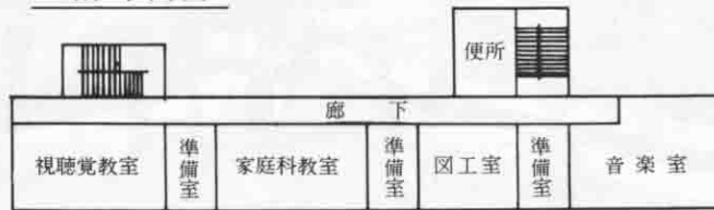
2階 平面図
