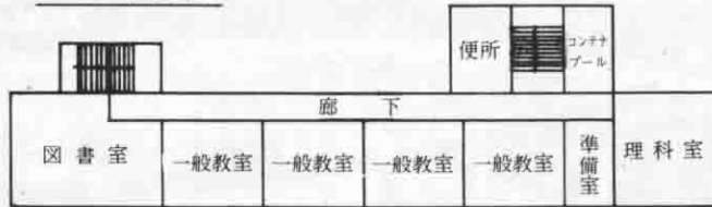
1階 平面図
