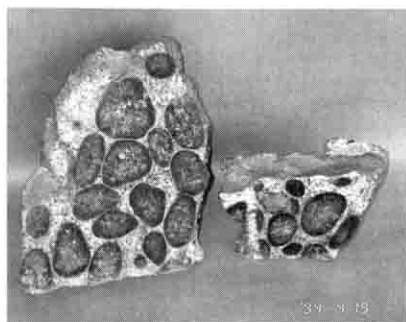
球状花崗岩の一部
