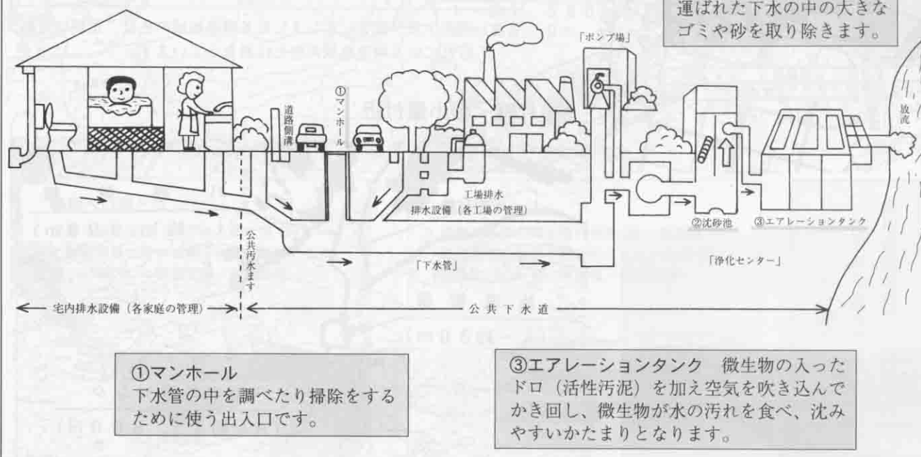
図-1 使った水を「キレイ」にするまで
