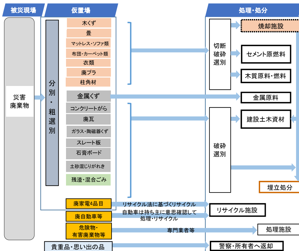
図表 3-7 災害廃棄物の種類別の処理方法（最大規模の場合）（例）
