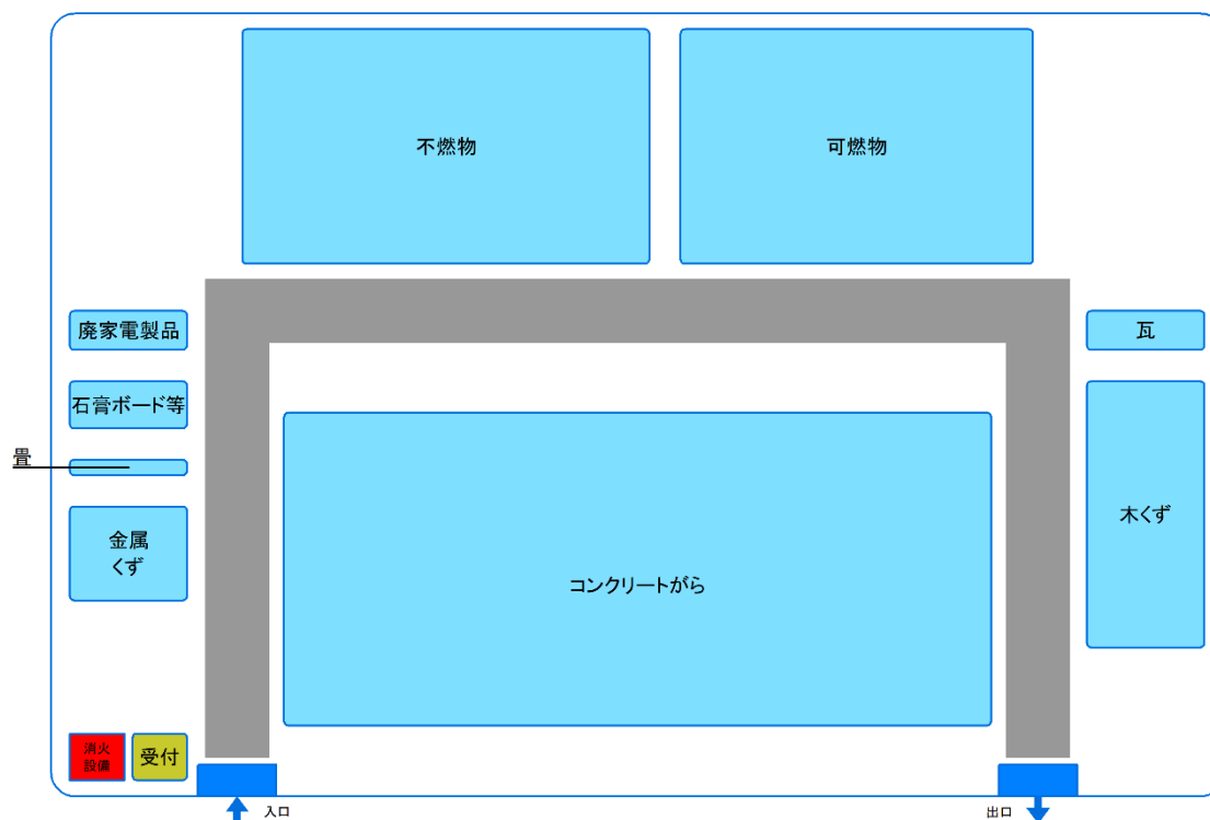
図表 3-12 一次仮置場の分別配置（例）
