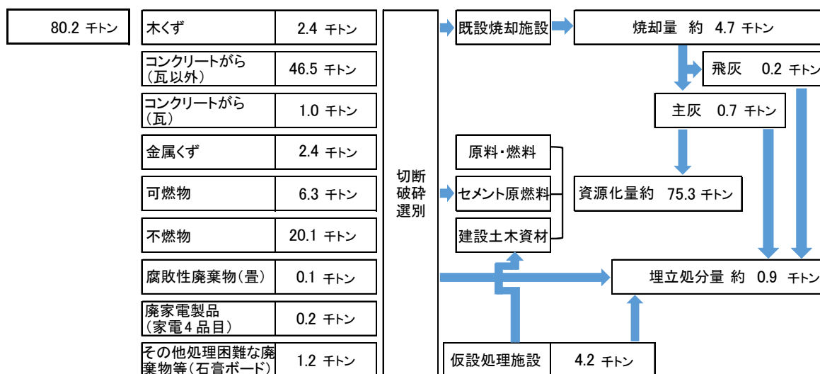
図表 3-16 災害廃棄物処理フロー（例）
