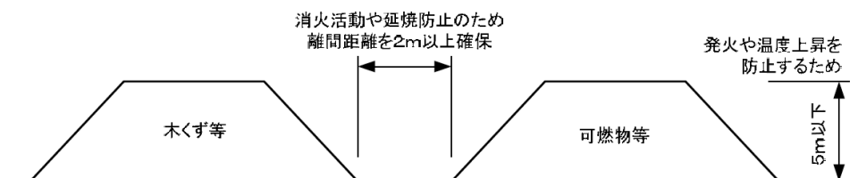
図表 3-22 可燃性廃棄物を並べて配置する場合
