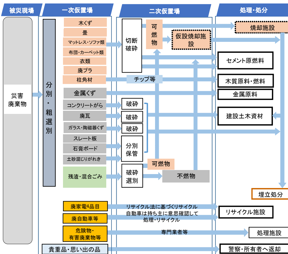
図表 3-7 災害廃棄物の種類別の処理方法（最大規模の場合）（例）
