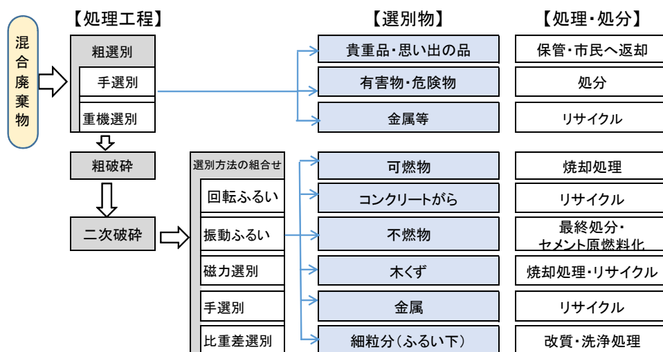
図表 3-14 混合廃棄物処理工程（例）
