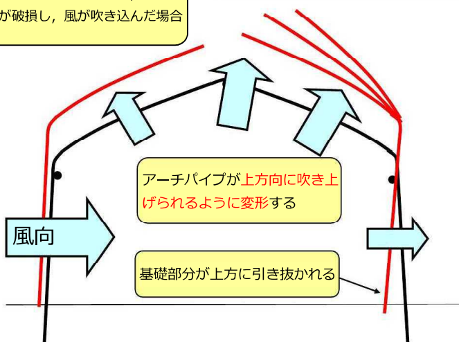
図-4 風の吹き込みにより内側から外側に破裂するパターン
